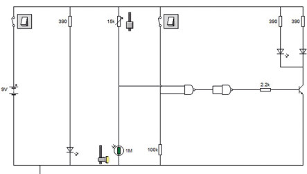
ΨΗΦΙΑΚΟ ΚΥΚΛΩΜΑ ΜΕ ΛΟΓΙΚΗ ΠΥΛΗ AND
