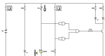
ΨΗΦΙΑΚΟ ΚΥΚΛΩΜΑ ΜΕ ΛΟΓΙΚΗ ΠΥΛΗ OR
