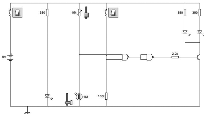
ΨΗΦΙΑΚΟ ΚΥΚΛΩΜΑ ΜΕ ΛΟΓΙΚΗ ΠΥΛΗ AND
