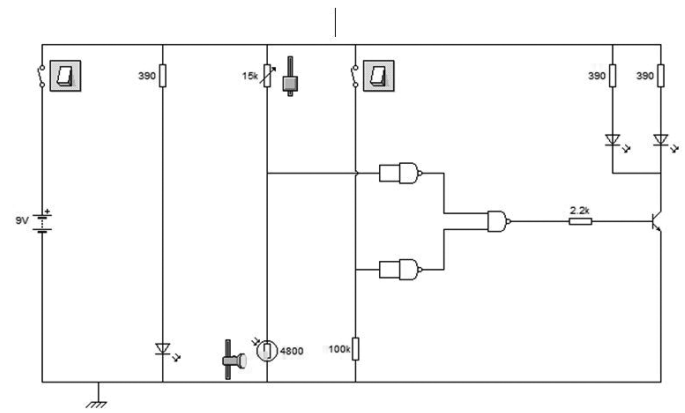
ΨΗΦΙΑΚΟ ΚΥΚΛΩΜΑ ΜΕ ΛΟΓΙΚΗ ΠΥΛΗ OR
